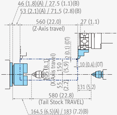
OD Holder
